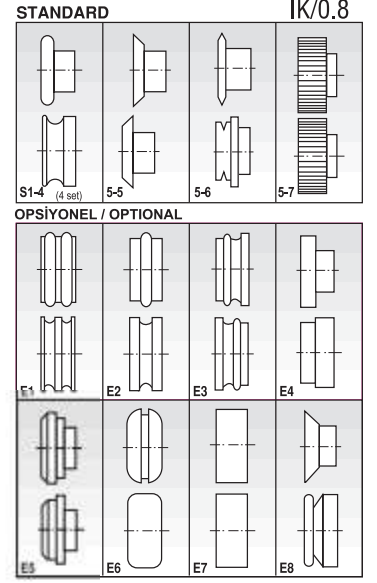
IK 0.8 7 takım standart vals topu ve top açma anahtarı ile beraber 7 set of standard rolls and roll key
